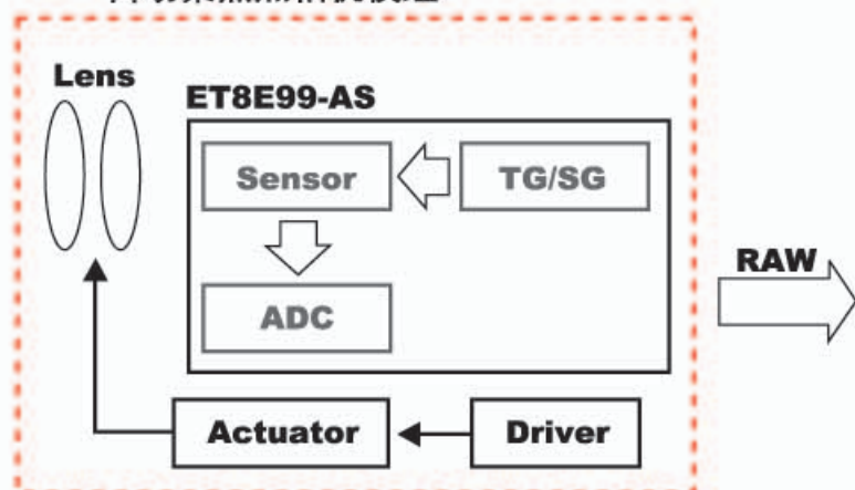
自动聚焦相机模组
